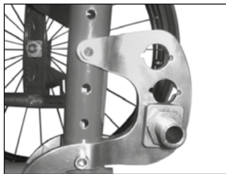
MG 86 Удлинение колесной базы
