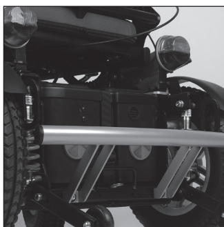
ЕА 62 Бампер
